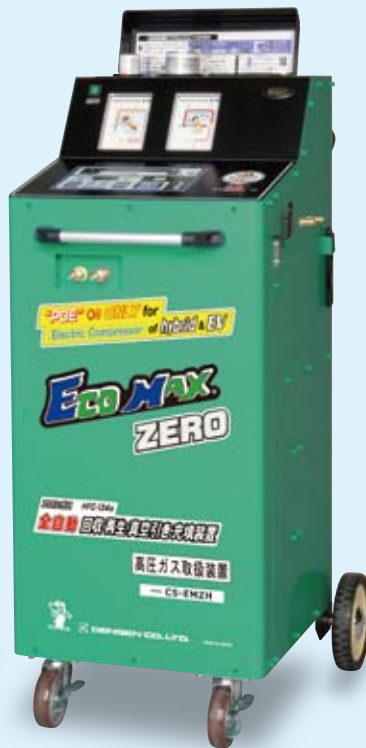
MODEL CS-EMZH プリンター無し(POE用)
